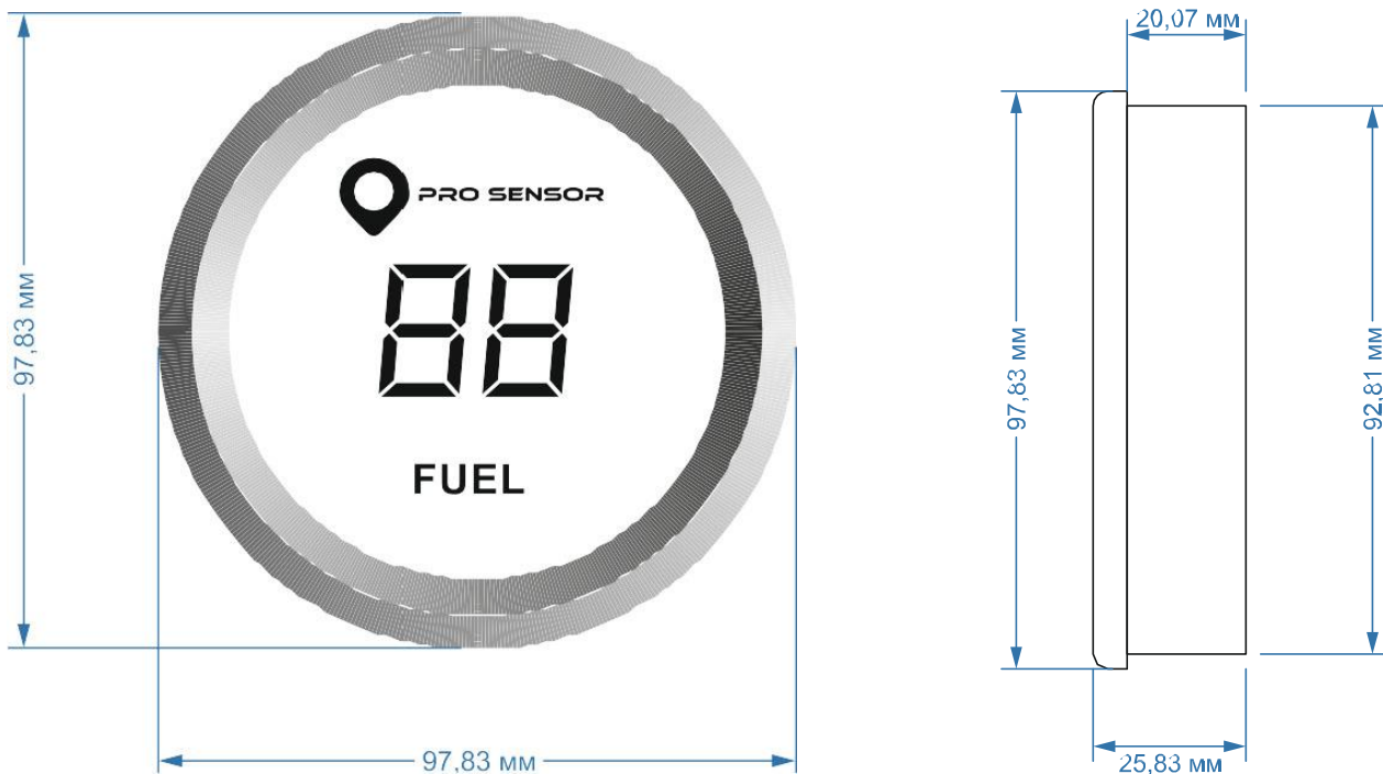
Рис. 2. Размеры индикатора уровня топлива. Место вывода кабеля может варьировать.
